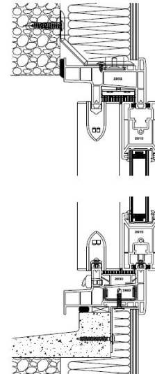
Isolation intérieure de 100 mm (possible de 70 à 180 mm)
