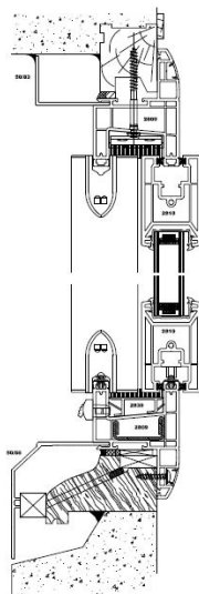
Ailette rénovation de 40 mm de série
