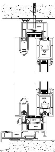
Pièce d'appui de 57 mm en base (possible en aile de 87 et 130 mm)
