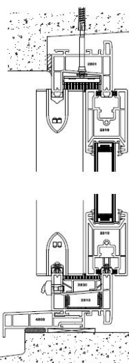
Dormant de 70 mm (avec ou sans ailette) et pièce d'appui de 57 mm en base
