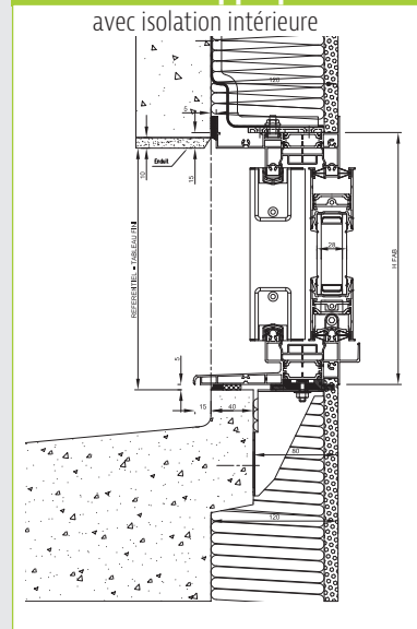
Possibilité de dormant monobloc 100/120/140/160 mm
