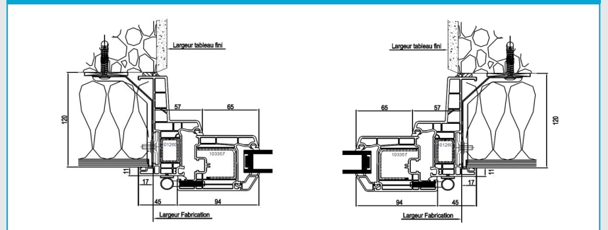
Isolation intérieure de 100 mm (possible de 70 à 180 mm)
