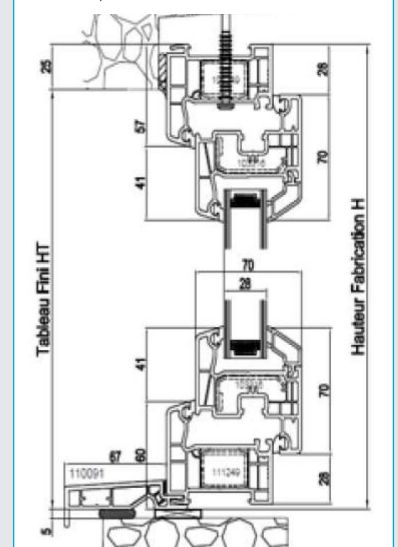
Dormant de 70 mm et pièce d'appui rapportée dépassant de 67 mm Disponible également en pose tunnel
