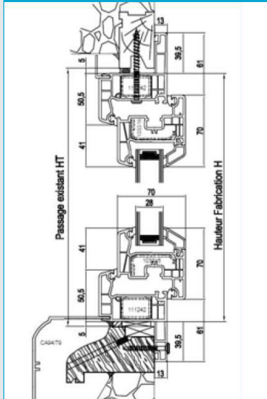
Ailette rénovation de 40 mm en base (possible en 60 mm en blanc)
