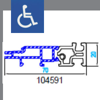
Seuil aluminium à rupture de pont thermique
