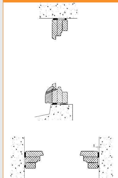
Dormant de 67 mm avec pièce d'appui (option couvre-joints)
